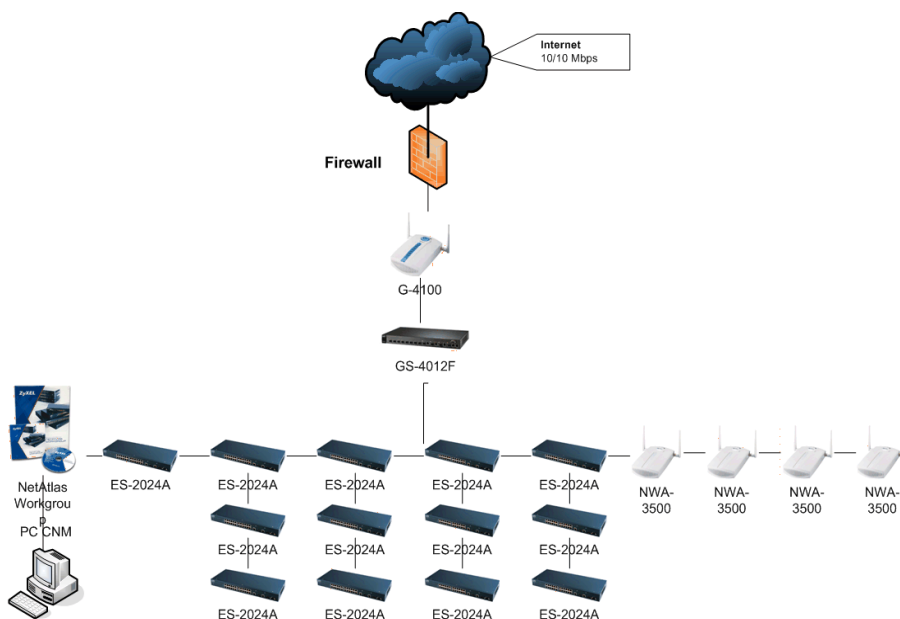
Obr.: Diagram sítě
